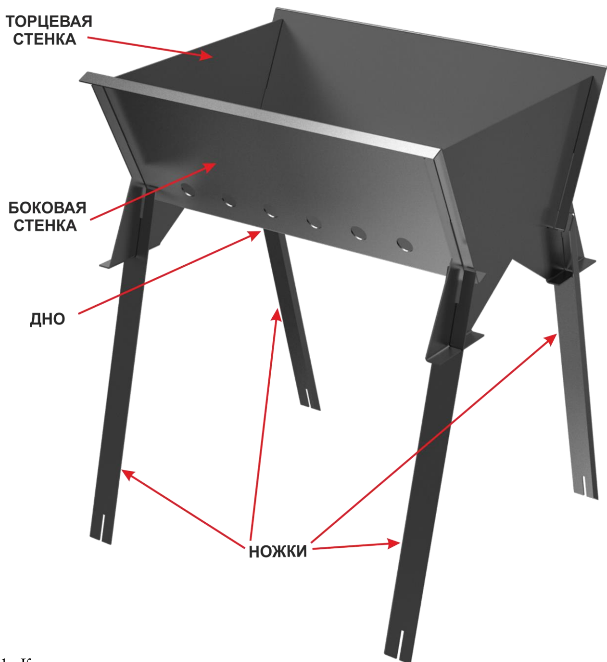
Рис. 1 Конструкция мангала
